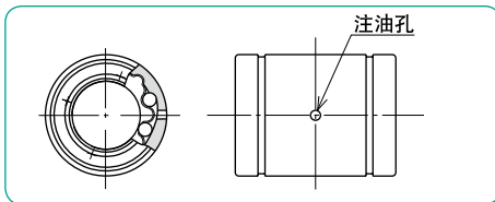
图C-8 注油孔规格—特殊规格—
