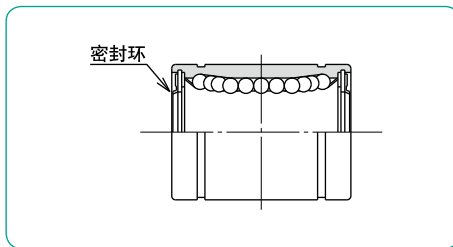
图C-10 双唇密封环形状
