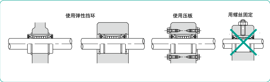
图C-3 标准型
