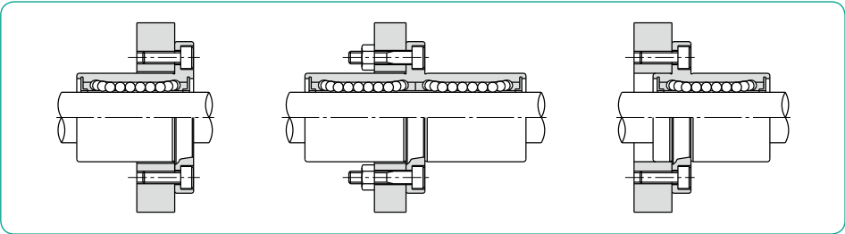
图C-6 法兰型
