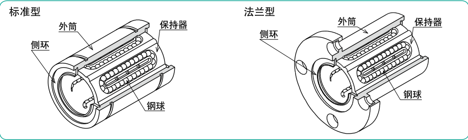
图C-1 NB直线轴承·衬套 (SM,KB,SW) 的基本结构
