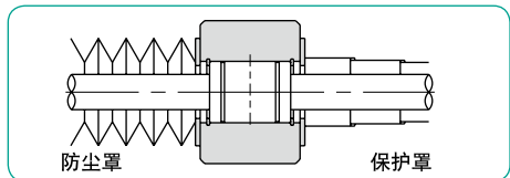
图C-11 防尘结构范例
