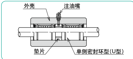
图C-8 注油孔规格—特殊规格—
