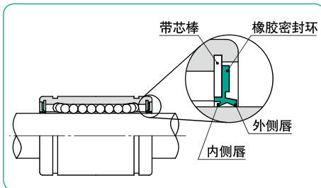
图C-10 双唇密封环形状
