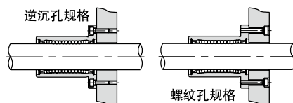
图C-14 特殊安装孔规格(例)
