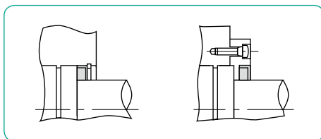
图C-13 毛毡密封环的安装范例
