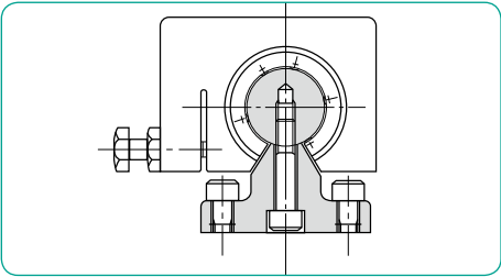
图C-5 开放型
