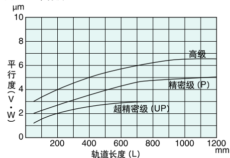
图G-5 平行度
