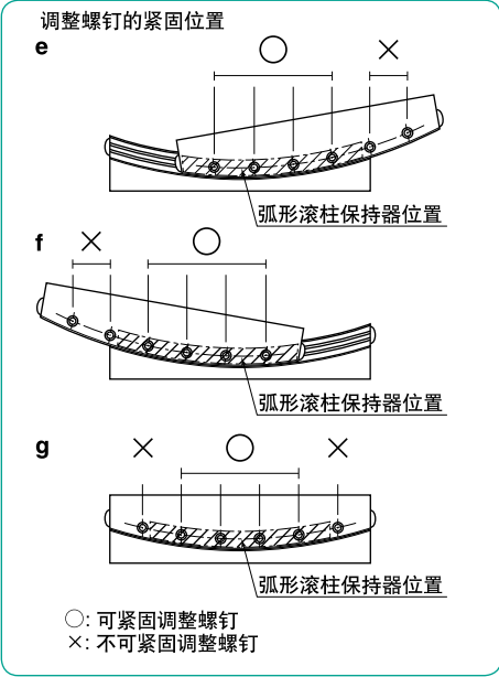
图G-41 安装方法(2)
