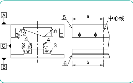
图G-34 安装面的精度
