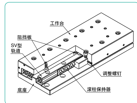
图G-18 SVT型的结构
