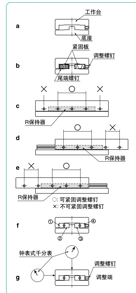
图G-13 安装方法
