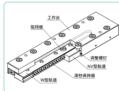
图G-19 SYT型的结构
