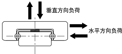
图G-24 负荷方向
