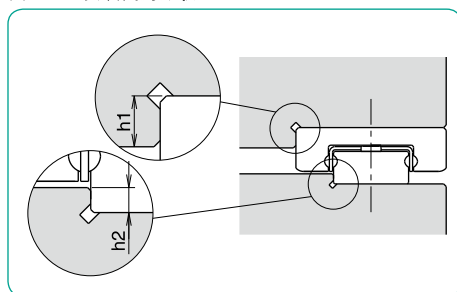
图G-26 安装面的形状-2
