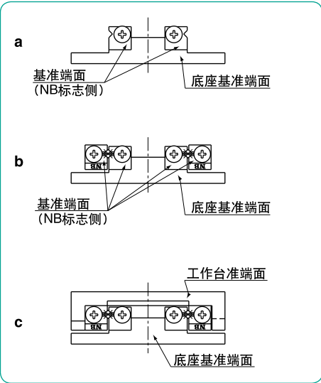
图G-36 安装方法(1)
