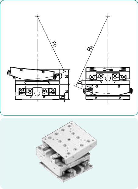
图G-42 2轴组合规格
