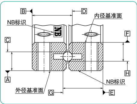
图G-33 精度的测量方法
