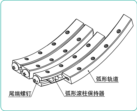
图G-31 RV型的结构
