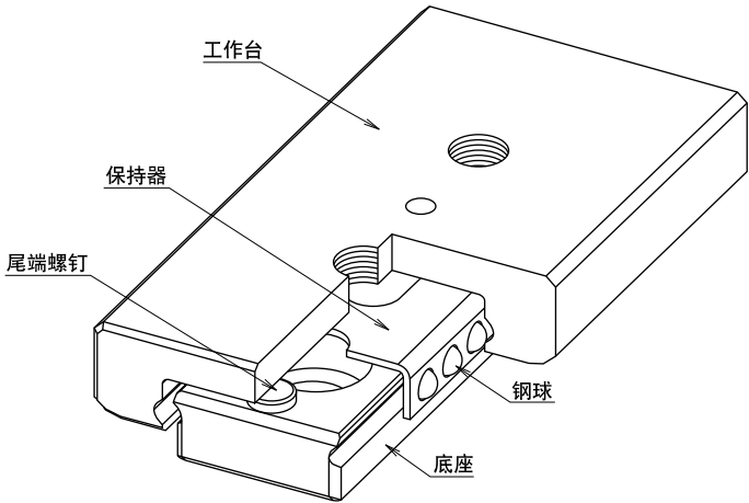
图G-22 SYBS型的结构
