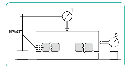
图G-20 精度的测量方法
