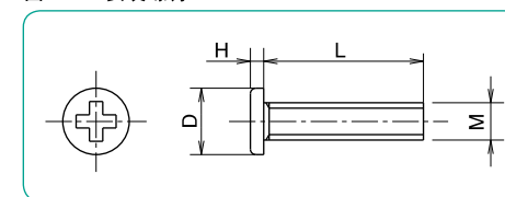
图G-29 安装螺钉
