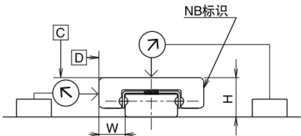
图G-23 精度的测量方法
