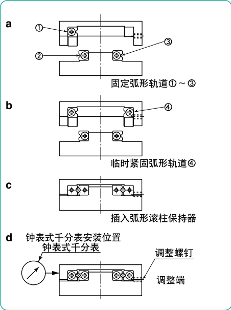
图G-40 安装方法(1)
