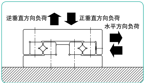
图G-7 负荷方向
