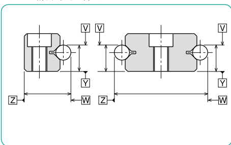
图G-6 精度的测量方法
