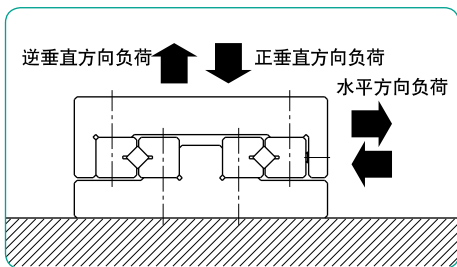
图G-21 负荷方向
