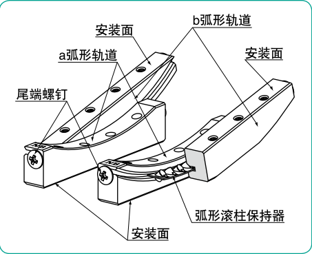
图G-30 RVF型的结构
