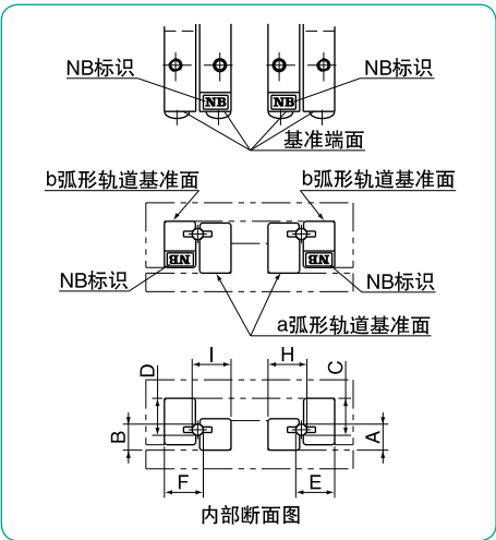
图G-32 精度的测量方法
